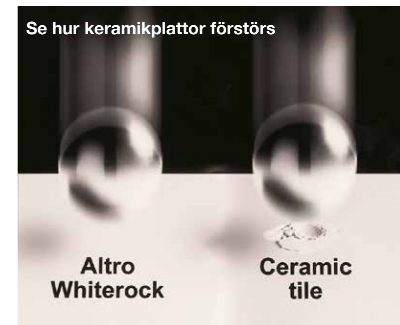
Stålkuletestet (BS EN438-2-1991)
