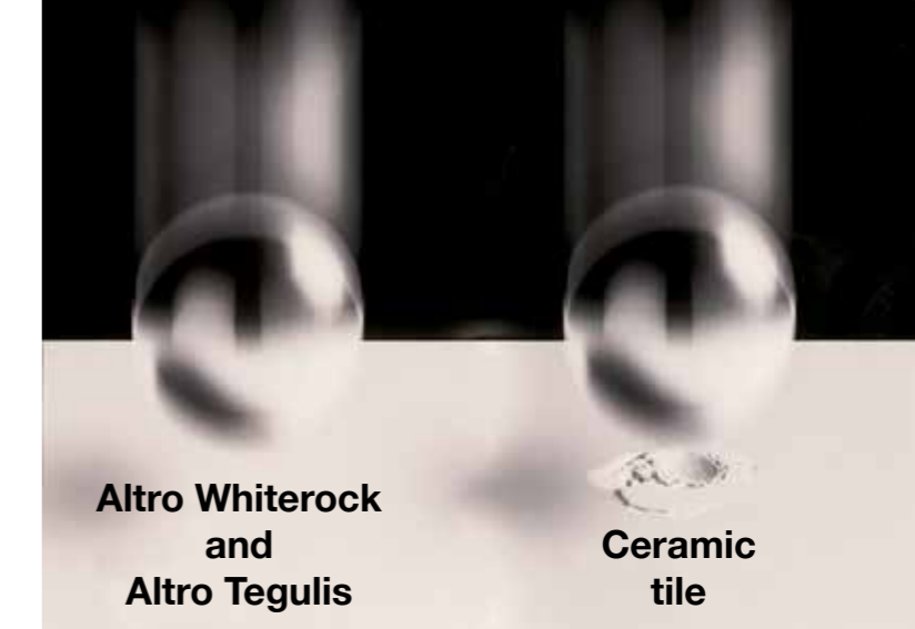
BS EN438-2-1991 Drop Ball Test
