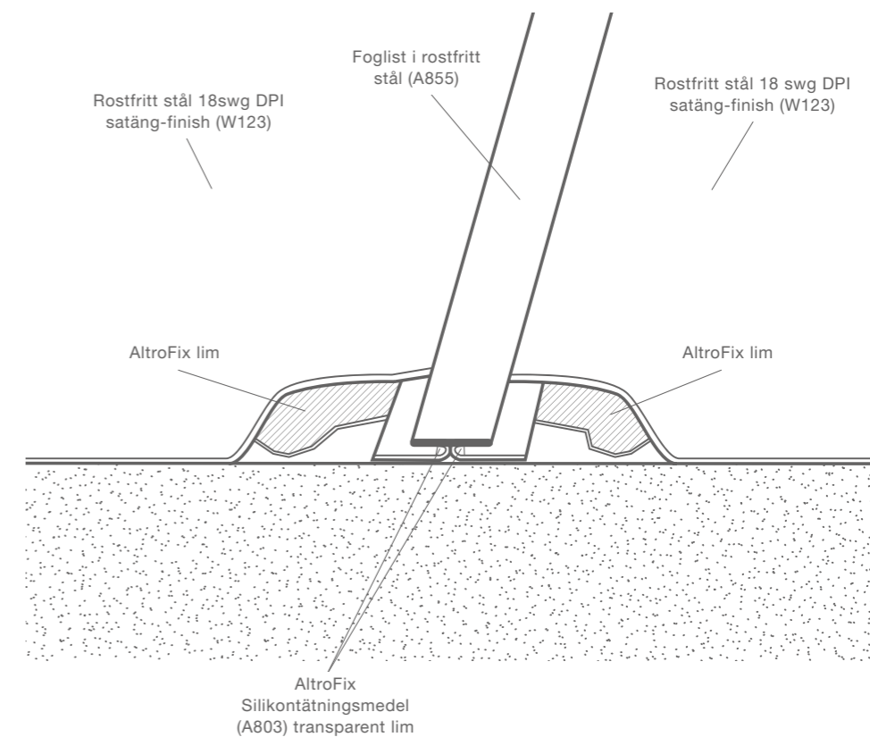
Altro Whiterock beklädnad i rostfritt stål till beklädnadsdetalj i rostfritt stål
