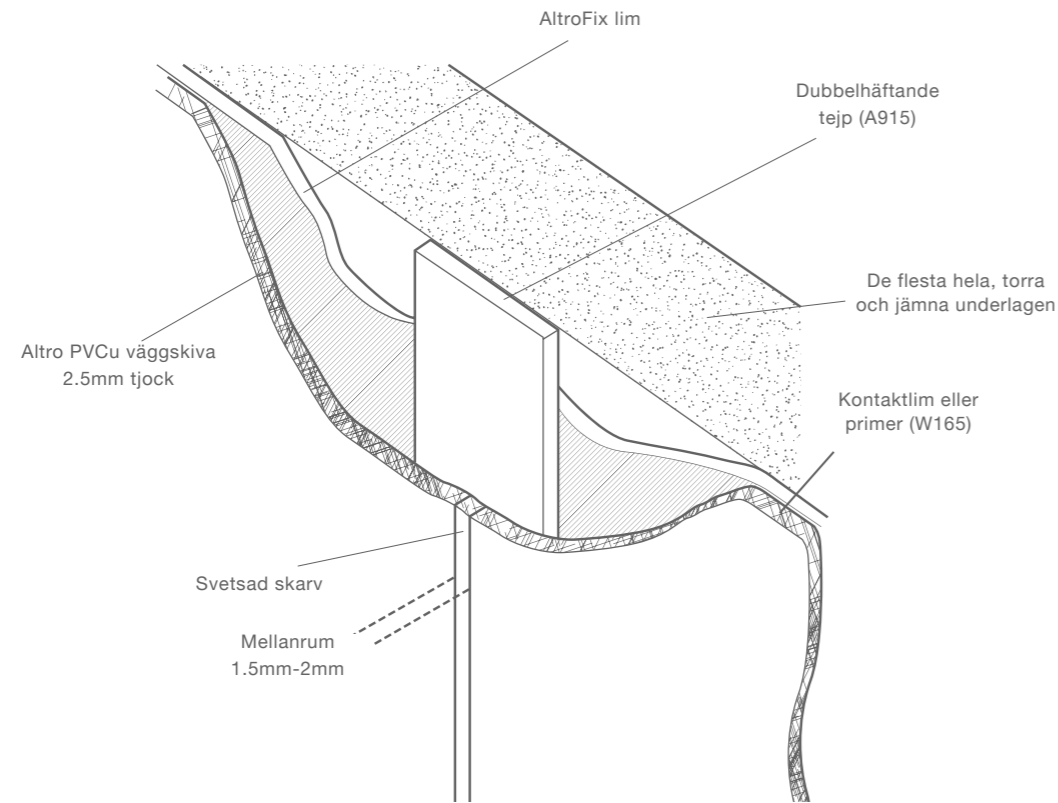
Altro Whiterock väggskiva till hartsgolvsdetalj
