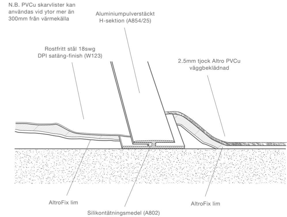
Altro Whiterock beklädnad i rostfritt stål till beklädnadsdetalj i rostfritt stål
