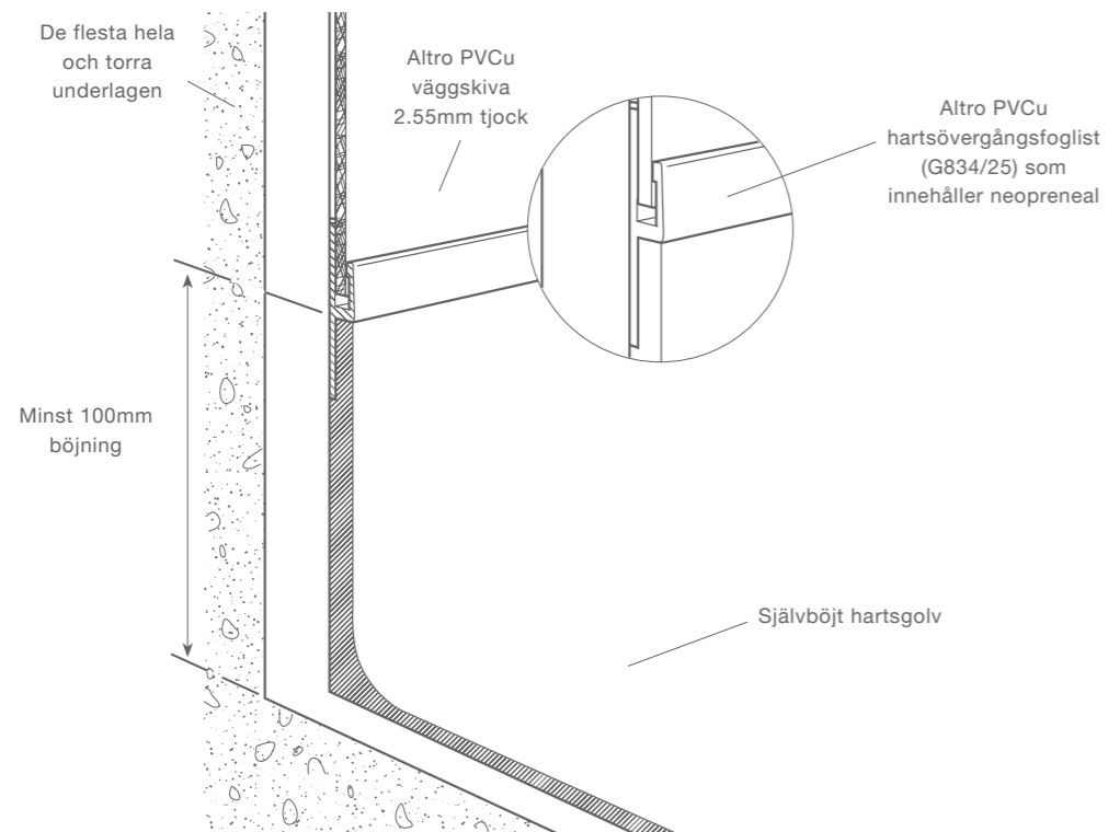
Altro Whiterock väggskiva till hartsgolvsdetalj
