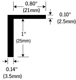
Altro gully angle - GA35/25
