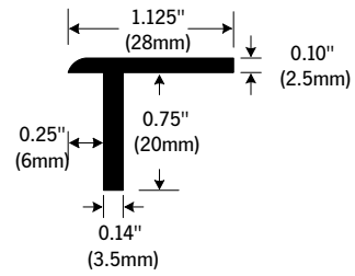
Altro gully edge - GE 25RE
