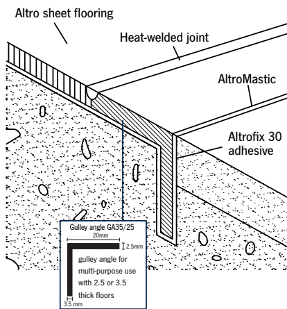
Altro gully angle - GA35/25
