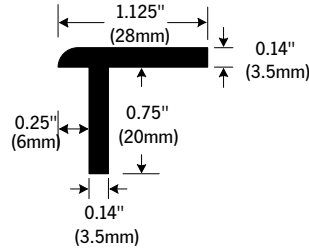
Altro gully edge - GE 35RE
