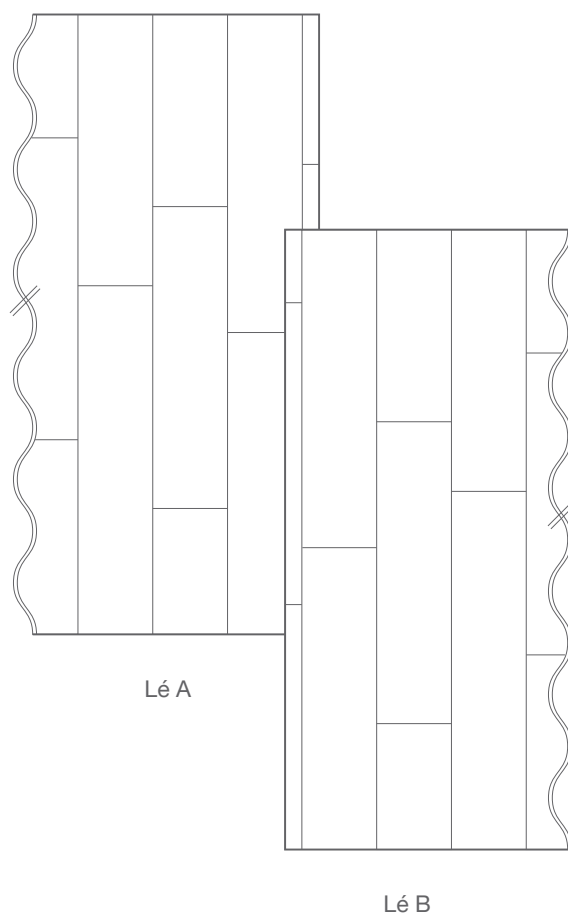
Schéma 2 – Les bords du lé ont une bordure étroite qui doit être recoupée pour obtenir une lame entière. Superposer le lé A sur le lé B selon les indications ci-dessus et couper le joint en coupant simultanément les deux lés de sorte que le joint soit positionné en bordure de lame.
